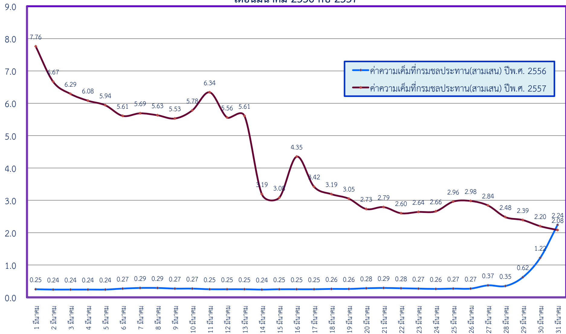
กราฟแสดงการเปรียบเทียบค่าความเค็มในแม่น้ำเจ้าพระยา ที่จุดตรวจวัดกรมชลประทาน(สามเสน) เดือนมีนาคม 2556 กับ 2557
